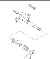
Schaltwelle & Schalthebel
