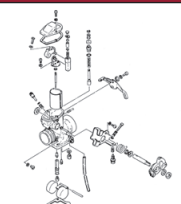
Vergaser
