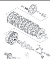
Kupplung
