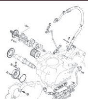
Ölpumpe & Ölfilter
