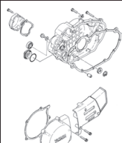
Kurbelgehäuse- deckel
