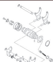
Schaltwalze & Schaltgabeln
