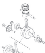
Kurbelwelle & Kolben
