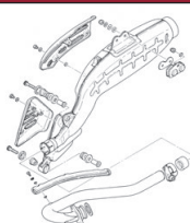
Auspuff
