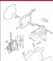
Seitendeckel & Werkzeugbox
