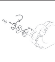
Unterbrecher & Fliehkraftregler
